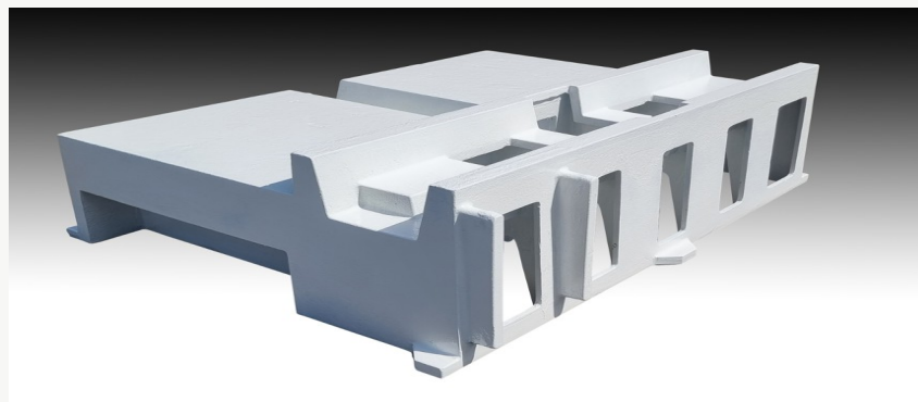
ベース鋳物 ・ FC300
