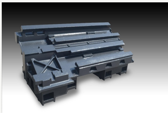
CNCベッド鋳物 ・ FC300
